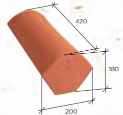
About de faîtière à sec grand cornet (départ) Réf. 826
