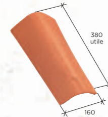
Faîtière sans emboîtement (2,5 par ml) Réf. 727 Crochet Réf. CR727
