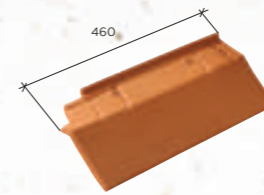
Bardelis "S" droit (2,7 par ml) Réf. 1052 (2)
